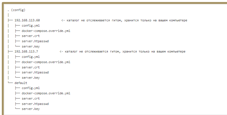
Рисунок 12 – Структура каталога config
