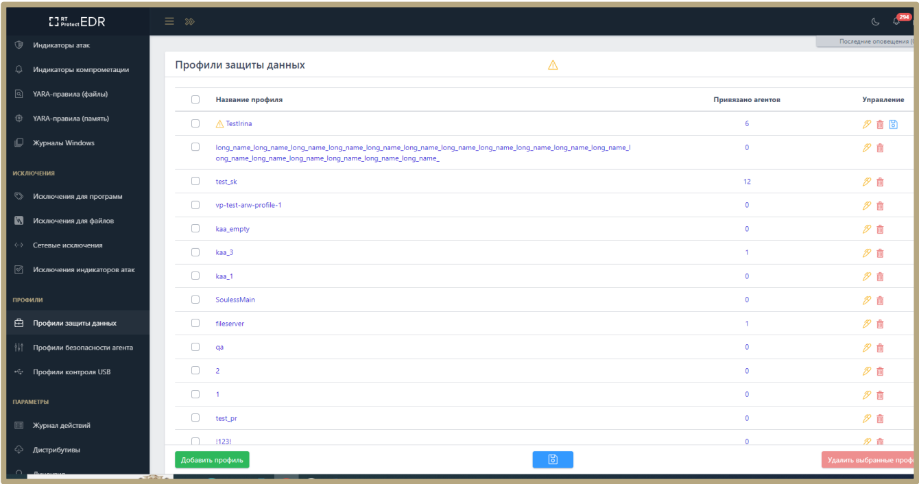
Рисунок 99 – Страница «Профили защиты данных»
