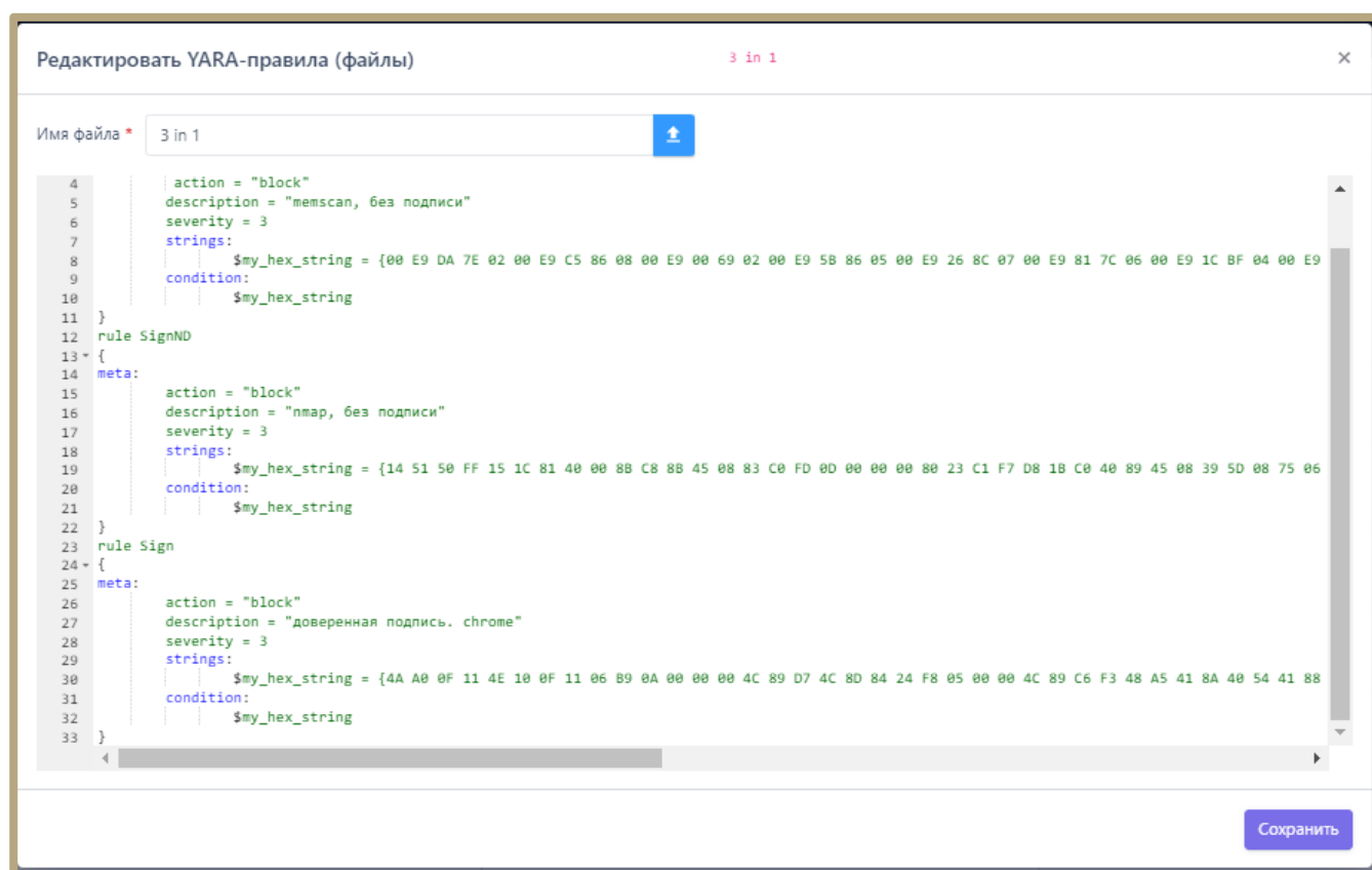
Рисунок 91 – Пример правила YARA
